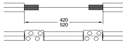
Схема підготовки кабелю для ремонтної муфти
