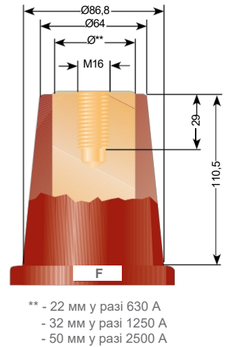
Бушинг із зовнішнім конусом "F" згідно з EN 50673
