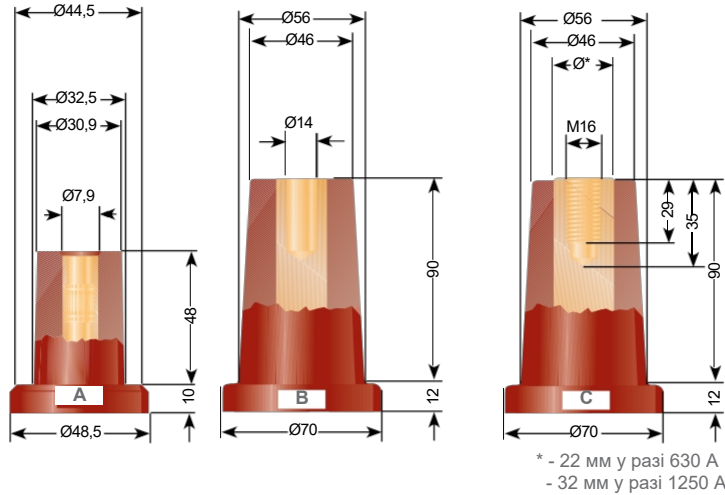
Бушинги із зовнішнім конусом "A", "B", "C" згідно з EN 50180 і EN 50181
