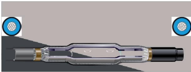
З'єднувальна муфта з інтегрованим металевим екраном і попередньо розтягнутою зовнішньою трубкою
