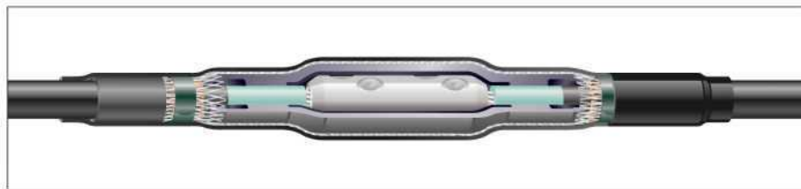
Соединительная муфта с отдельным металлическим экраном экраном и наружной трубкой Rayvolve
