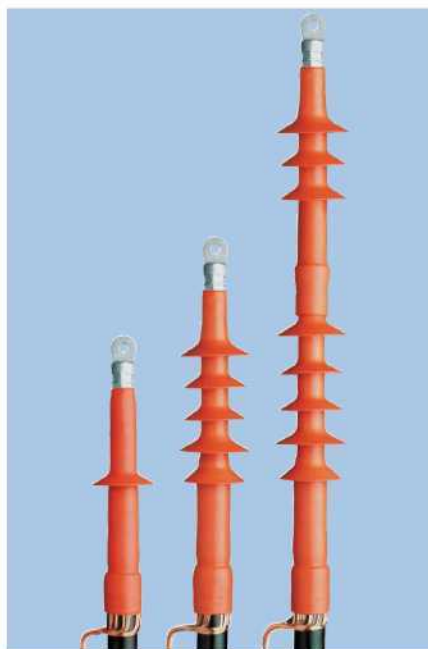
Муфты наружной установки
